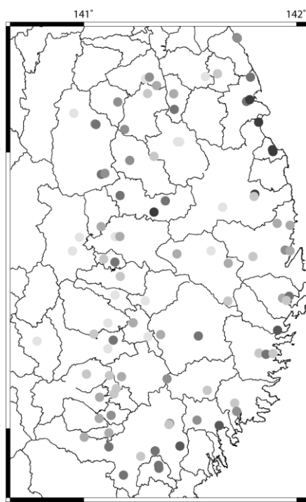
図8 震度増幅 ( V_s700\text{m/s} 以上)
