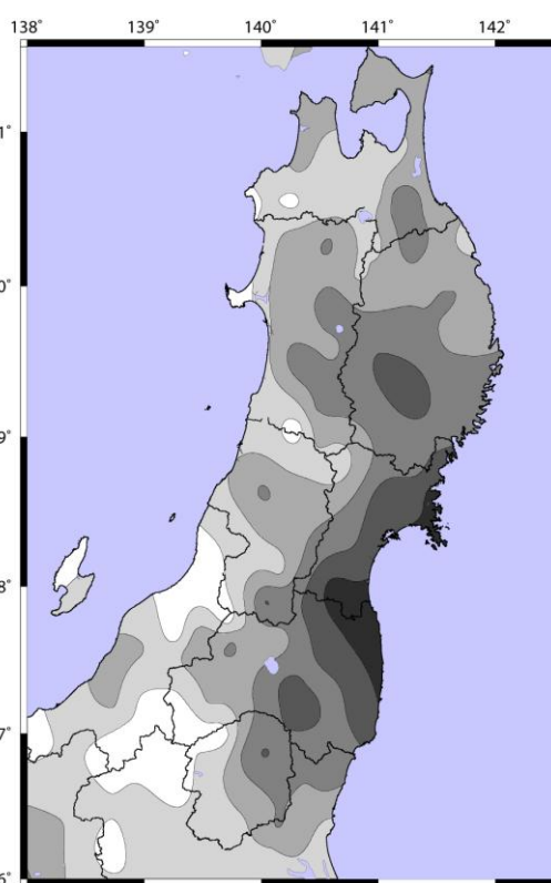
図6 地中震度分布 ( V_s700\text{m/s} 以上)
