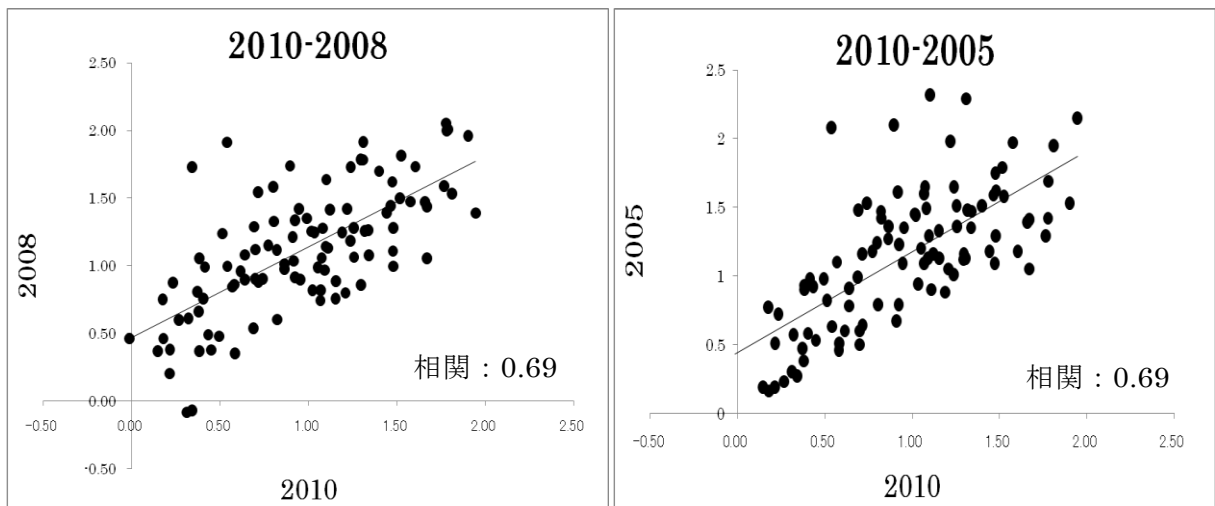
図 1 2 2010-2008 の震度増幅の相関
