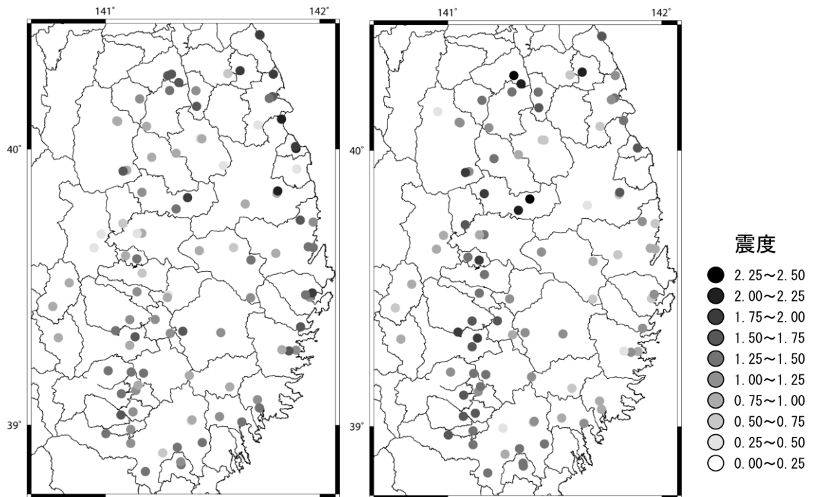
図 1 0 2008 年岩手・宮城内陸地震の震度増幅
