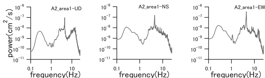
図2 111018_A2_area1のUD, NS, EW成分のパワースペクトル
