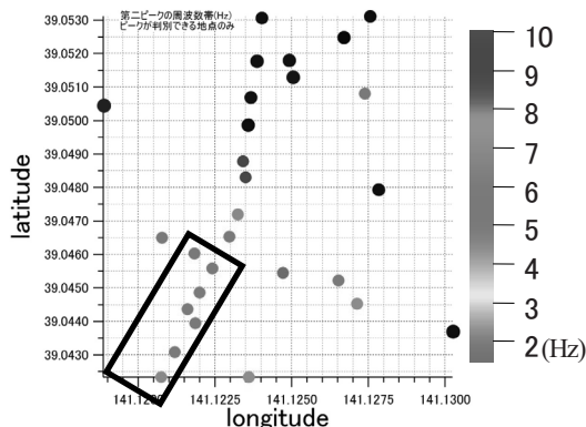
図4 H/V の第2 ピーク卓越周波数
