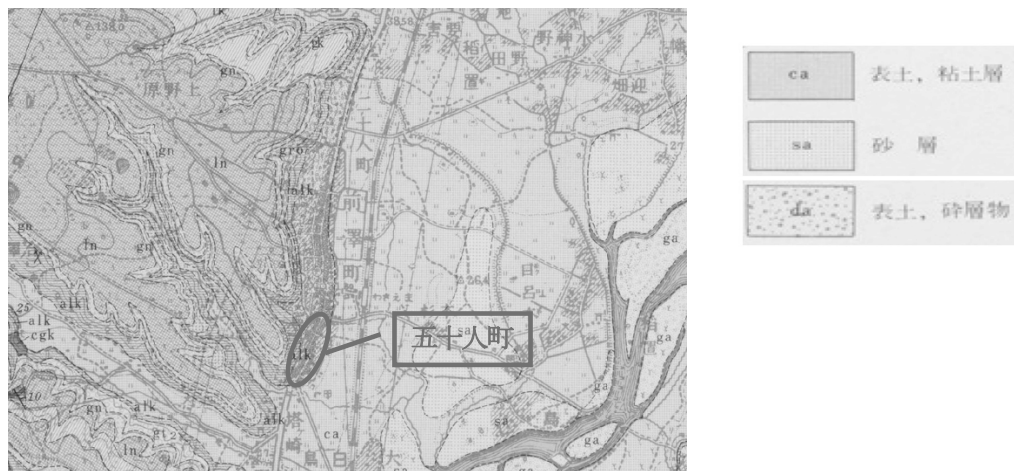
図11 前沢区における5万分の1表層地質図(国土交通省)
